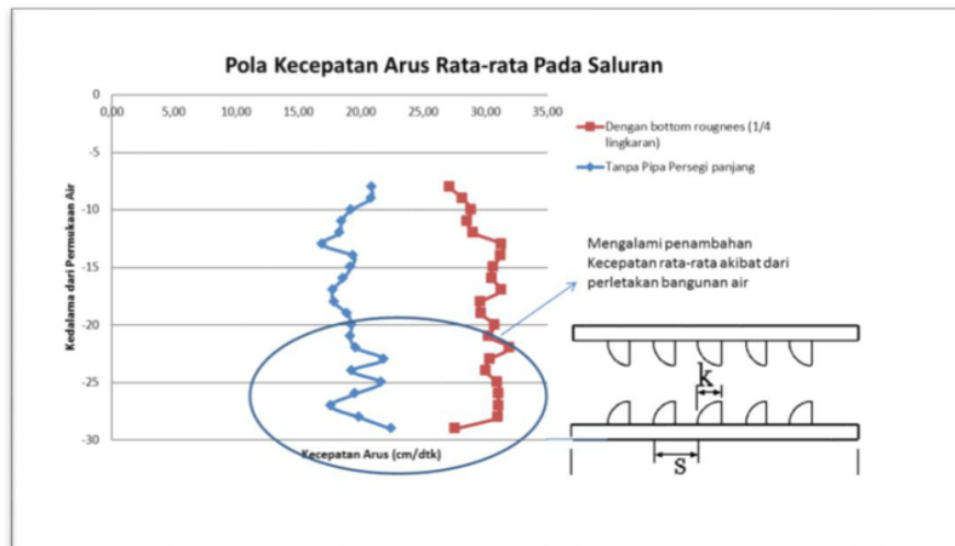
Gambar 4. Gambar Pola Kecepatan Arus Rata-rata pada Salauran
