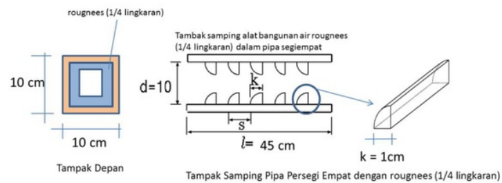
Gambar 2. Gambar dan foto Saluran Dua Dimensi Tampak Samping
